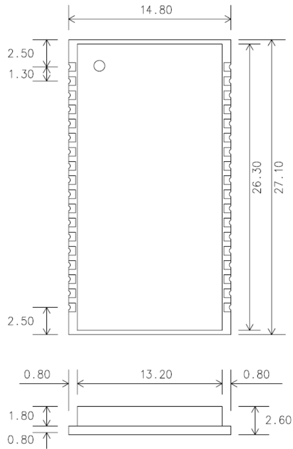
그림 1-3 모듈 치수
