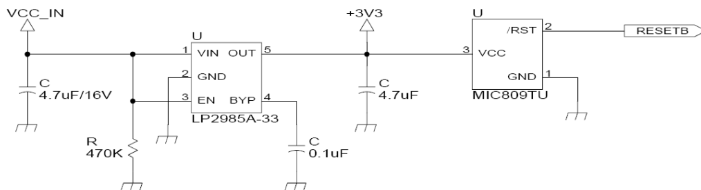
[전원 인터페이스]
